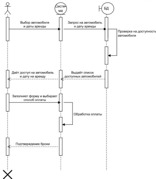
Рисунок 2 – Диаграмма последовательностей
